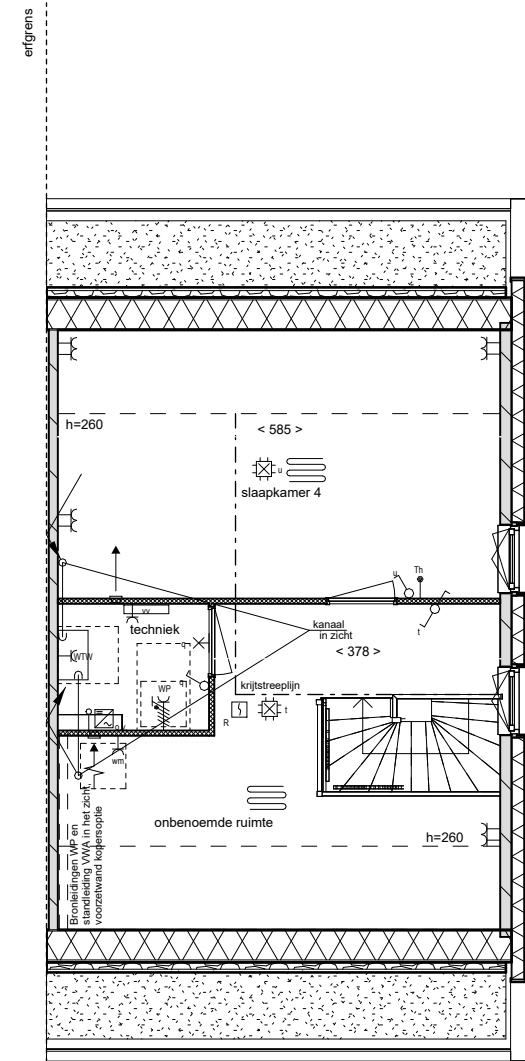
02 tweede verdieping
