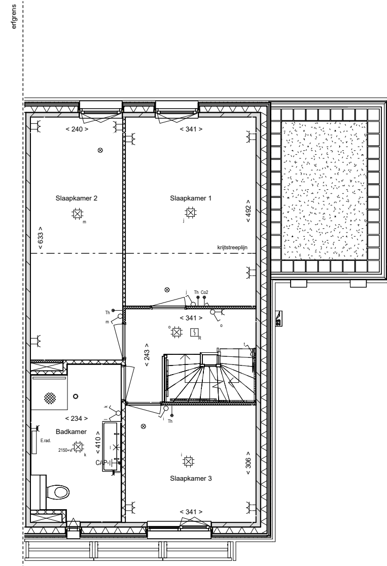
01 eerste verdieping
